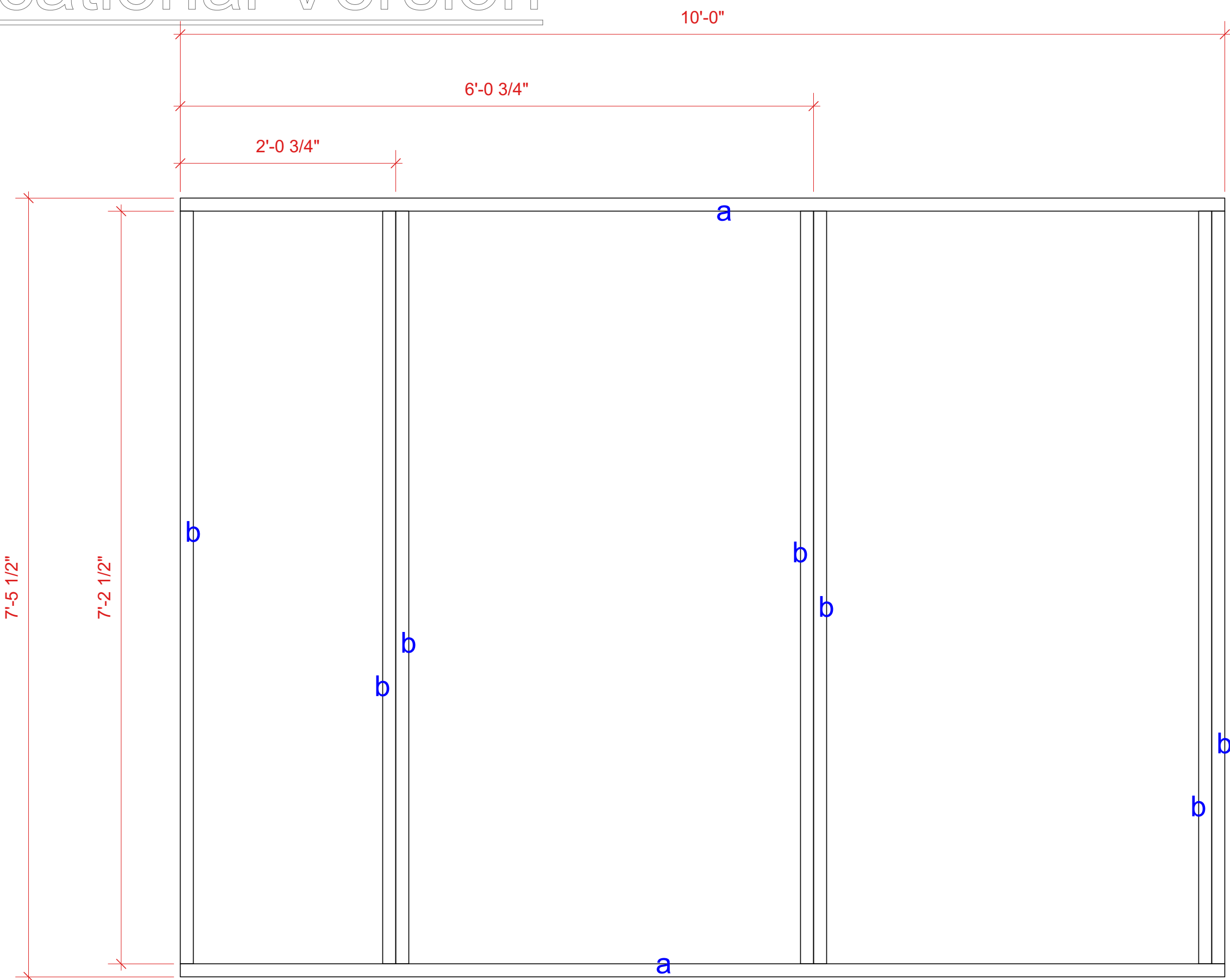
3 BACK STUD WALL C Scale: 1" = 1'-0"
