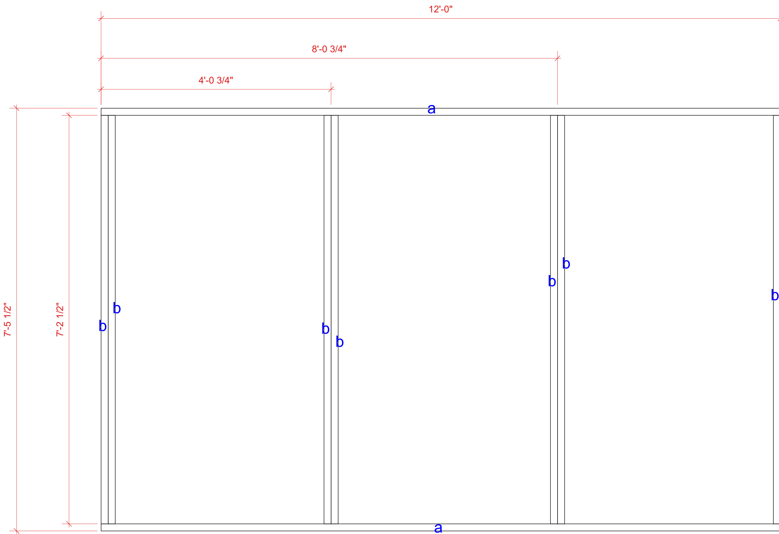
1 BACK STUD WALL A Scale: 1" = 1'-0"
