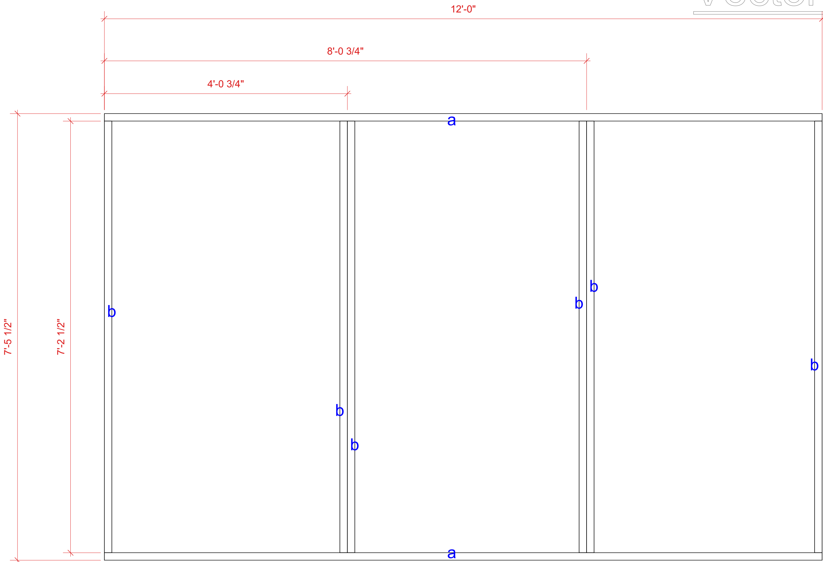
2 BACK STUD WALL B Scale: 1" = 1'-0"
