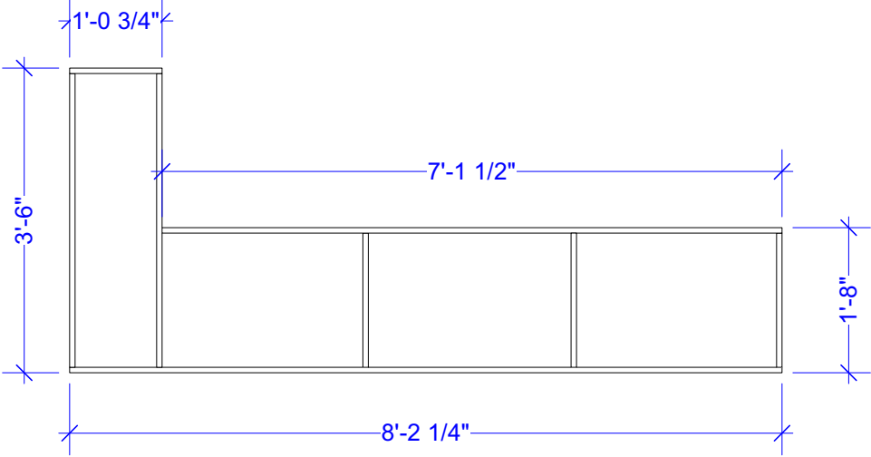
1 WALL G Scale: 1/2" = 1'-0"
