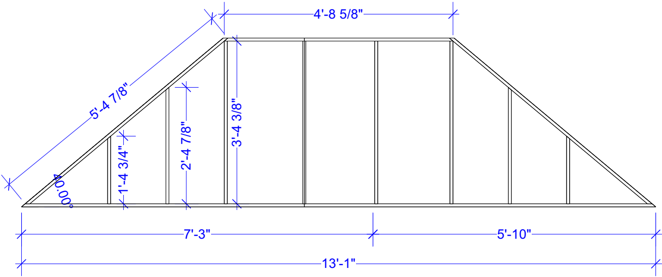
1 HEADER E Scale: 1/2" = 1'-0"
