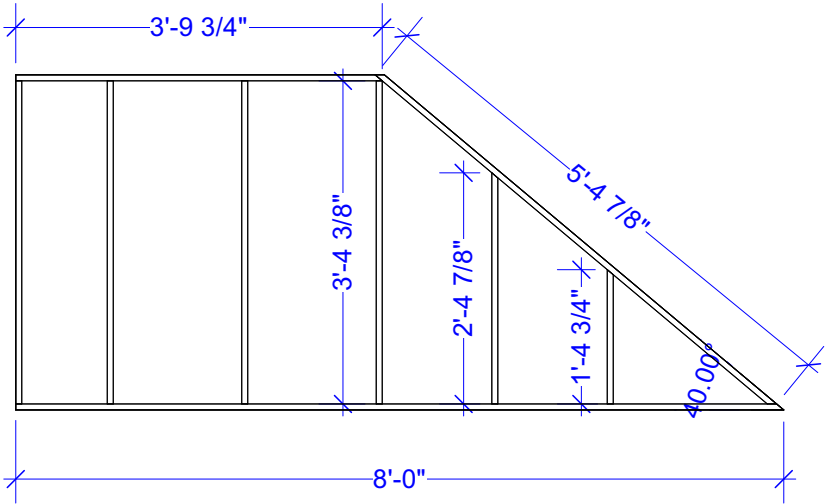
2 HEADER C2 Scale: 1/2" = 1'-0"
