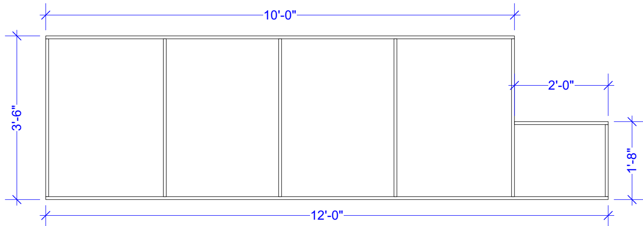
2 WALL B Scale: 1/2" = 1'-0"
