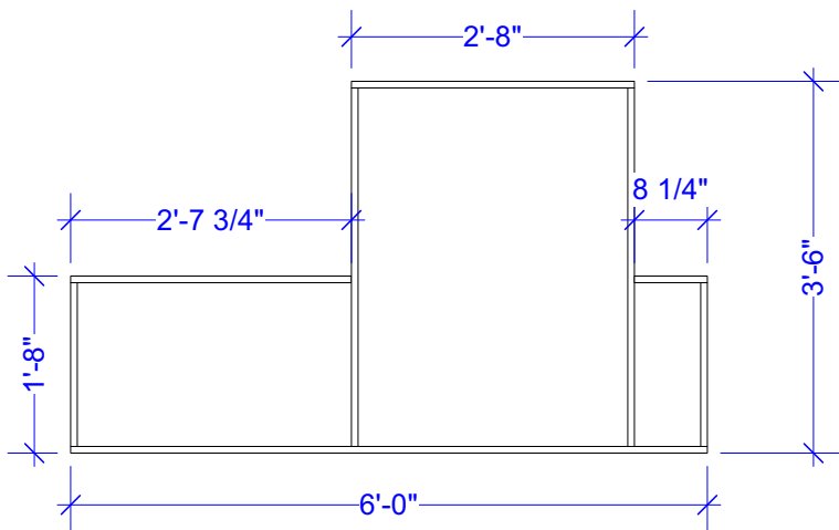
1 WALL F Scale: 1/2" = 1'-0"
