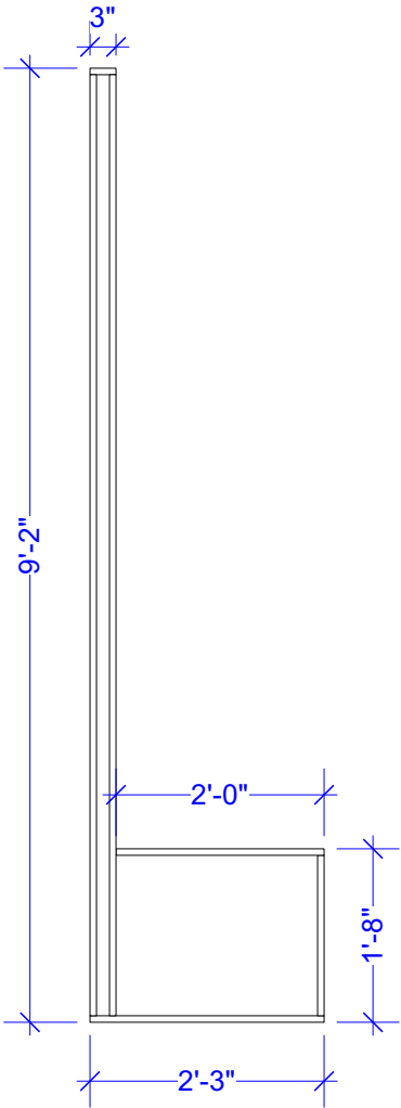
2 Scale: 1/2" = 1'-0" WALL L
