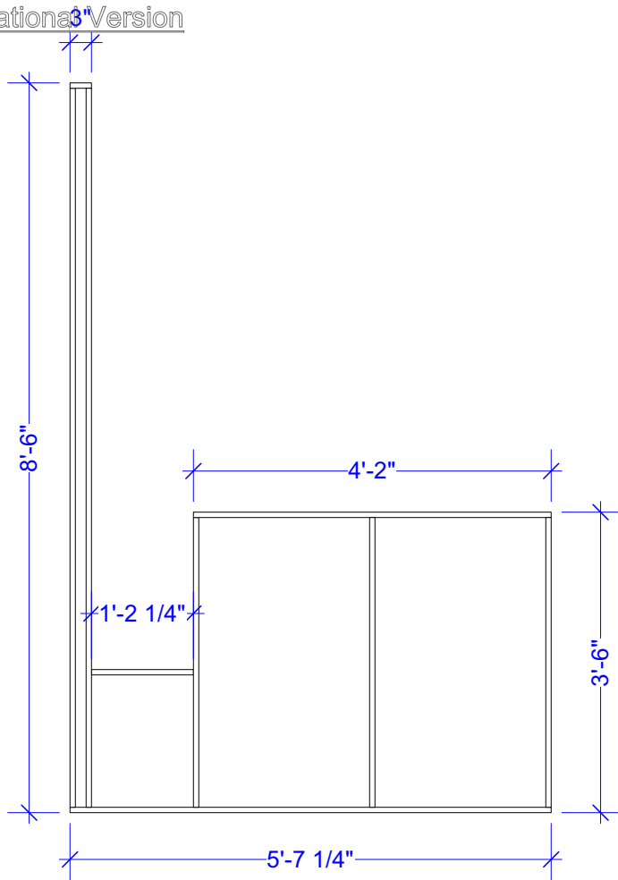
2 WALL E Scale: 1/2" = 1'-0"
