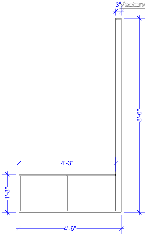
8 WALL D Scale: 1/2" = 1'-0"
