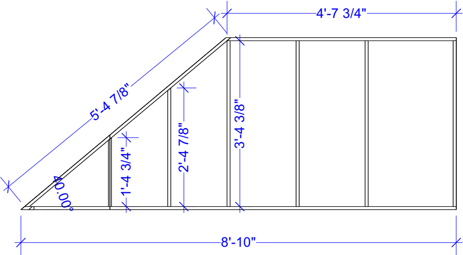
1 HEADER C1 Scale: 1/2" = 1'-0"
