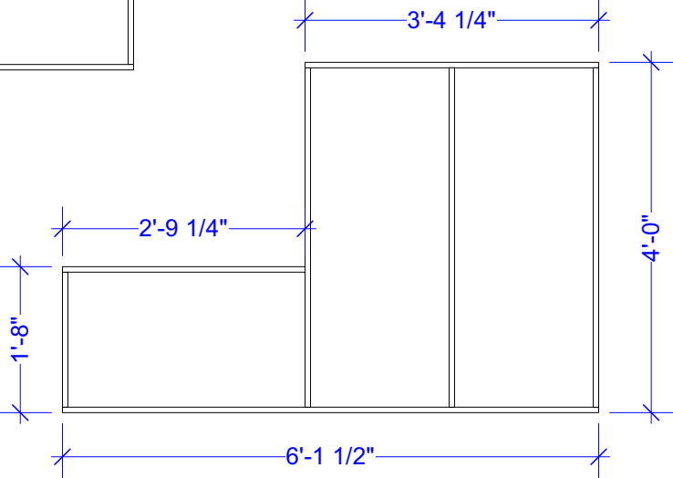
5 WALL O Scale: 1/2" = 1'-0"
